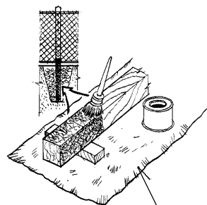
ПОЛИЭТИЛЕНОВАЯ ПЛЕНКА
