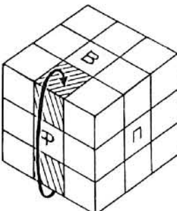
A10 L^{-1} P \Phi^2 L P^{-1} H^2 \Phi \dot{n} \rightarrow \Phi \delta
