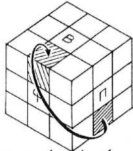
A9 L^{-1} P \Phi^{-1} L P^{-1} H \dot{n} n \rightarrow \Phi \delta
