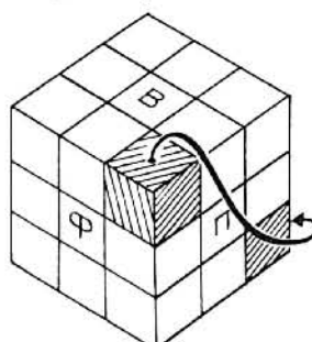
A8 \Phi H^2 \Phi^{-1} H^{-1} \Phi \delta n \rightarrow n H \dot{\tau}
