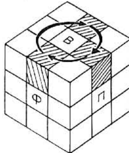
A11 P^2 H^{-1} L^{-1} P B^2 L P^{-1} \Phi^2 H P^2 \begin{cases} \Phi \delta \rightarrow \tau \delta \rightarrow n \delta \rightarrow \Phi \delta \\ \dot{\phi} b \rightarrow \dot{\tau} b \rightarrow \dot{n} b \rightarrow \dot{\phi} b \end{cases}
