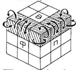
A12 \Phi B \Phi^2 L \Phi L^2 B L B^2 \begin{cases} \dot{\phi} b l \rightarrow \Phi \delta l \rightarrow \Phi b l \rightarrow \dot{\phi} b l \\ \dot{\phi} b n \rightarrow \Phi \delta n \rightarrow \Phi b n \rightarrow \dot{\phi} b n \\ \dot{n} t b \rightarrow n t b \rightarrow n t \delta \rightarrow \dot{n} t b \\ \dot{\phi} b \rightarrow \Phi \delta \rightarrow \dot{\phi} b \\ \dot{n} b \rightarrow n \delta \rightarrow \dot{n} b \end{cases}
