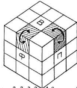
A6 P^2 \Phi^2 P^2 \Phi P B^2 P B \Phi P B \Phi B^2 \Phi^{-1} \dot{\phi} b \rightarrow \Phi \delta
