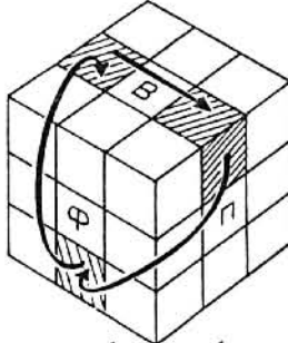
A5 B P^{-1} L \Phi^2 P L^{-1} B \begin{cases} \dot{\phi} n \rightarrow \delta l \rightarrow \delta n \\ \delta n \rightarrow \dot{\phi} n \end{cases}
