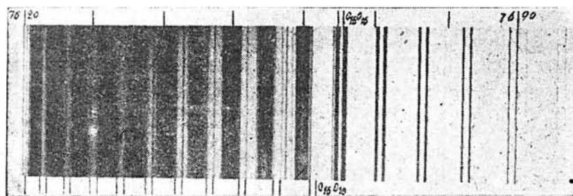
Рис. 11. Инфракрасный спектр кислорода.
