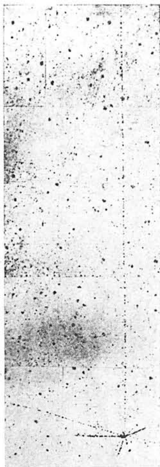
Рис. 12. Фотография следов, оставленных летящими осколками атомного ядра в слое фотопластинки.
